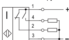
Схема подключения индуктивной нагрузки
