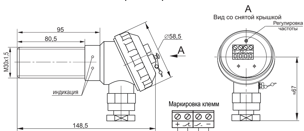
Габаритный чертёж
